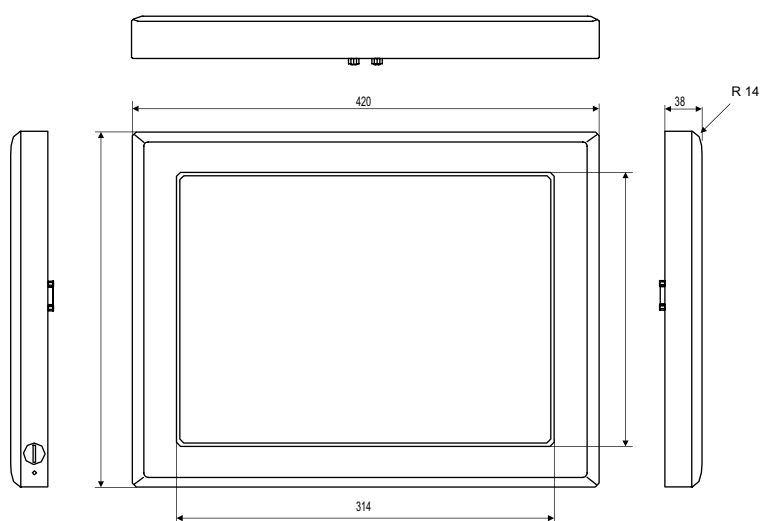
Наружные размеры 5D5212.04
